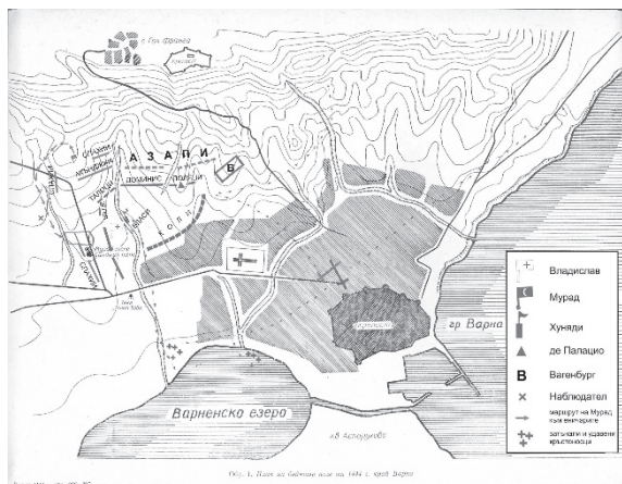
Фиг. 3. Скица на битката от 1444 г. край Варна върху карта на Георги Джингов от 1964 г.
